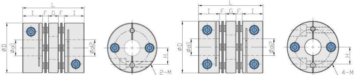
外徑 \phi 27 \sim \phi 34
