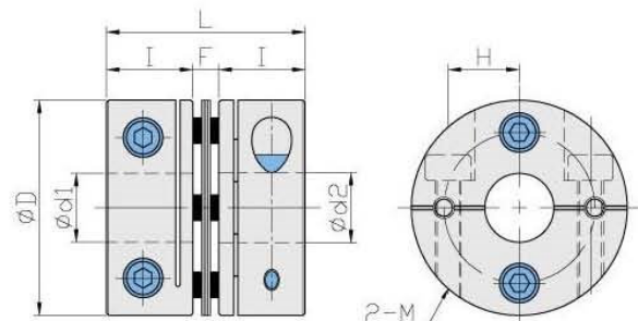
外徑 \phi 40 \sim \phi 65
