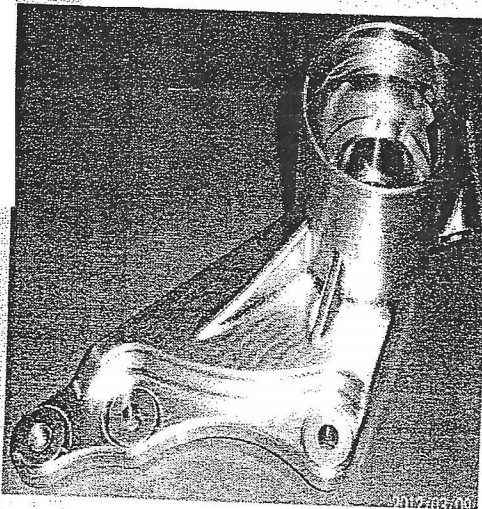
沙灘車零件 曲面加工
