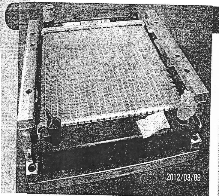
沙灘車水箱治具設計製作
